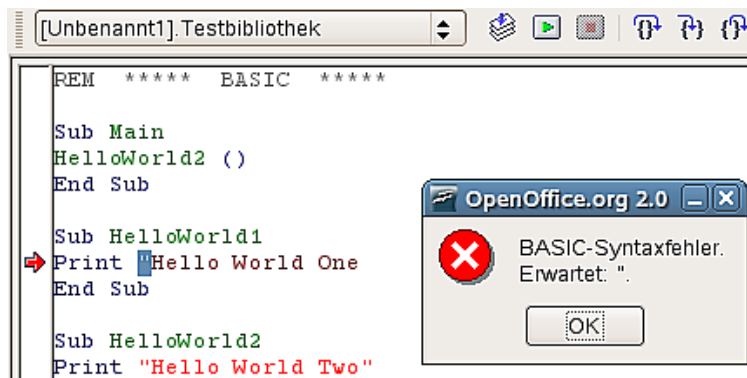
Abbildung 13: Makro mit Fehlermeldung
