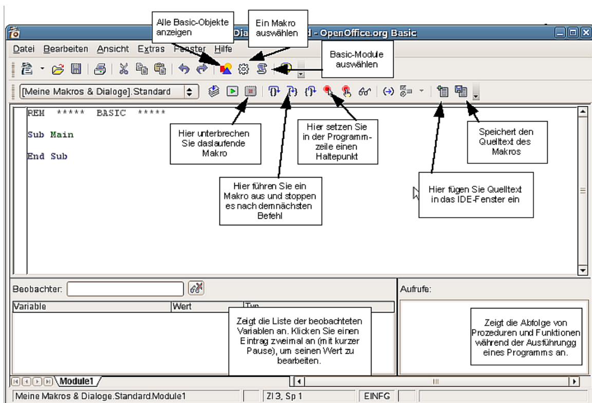
Abbildung 15: Die wichtigsten Elemente der IDE
