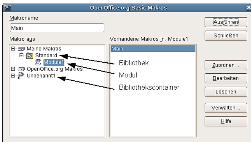
Abbildung 1: Verwaltung von Makros und Bibliotheken
